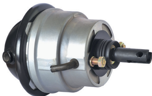
Kombibremszylinder, Keilbremse Brake Cylinder, wedge brake
